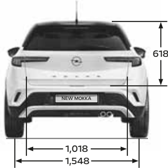
המידות במ"מ
